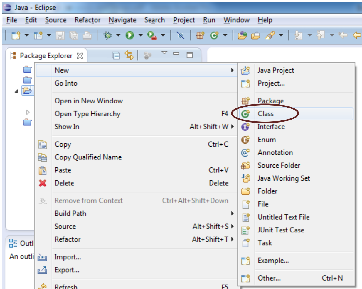
Gambar 5 Buat kelas
